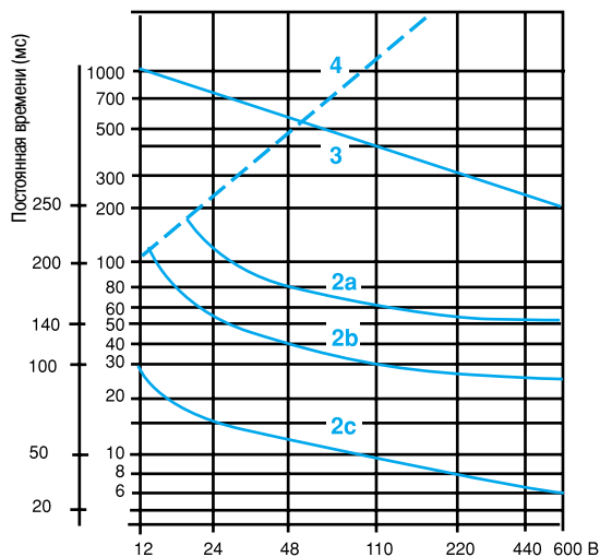
Мощность размыкания (Bt)
